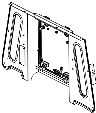
RE R P NEL SSEMBLY P/N:8SV-106-00001
