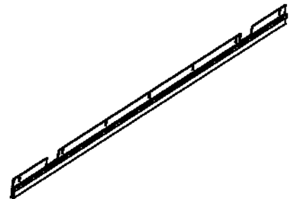
C-PILLAR BRACKET (2 PER CAB) P/N: 8SV-110-00020
