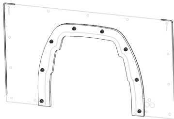
DOOR ASSEMBLY, RIGHT P/N: 8SV-107-00048-R
