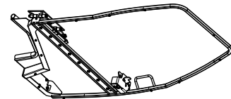
DOOR FRAME ASSY, RIGHT, NO SKIN P/N: 8SV-YDGR-RDF-NS
