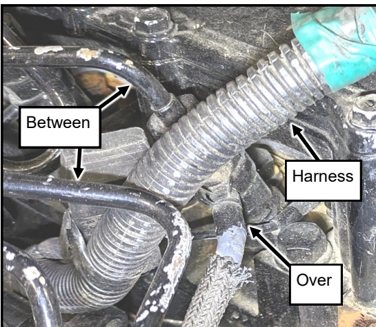
Fig. 1.33b (Route Wires)
