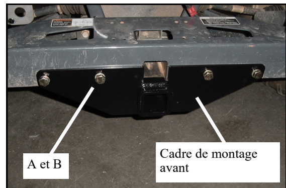
Fig 2.1 Montage de la plaque d'attelage avant
