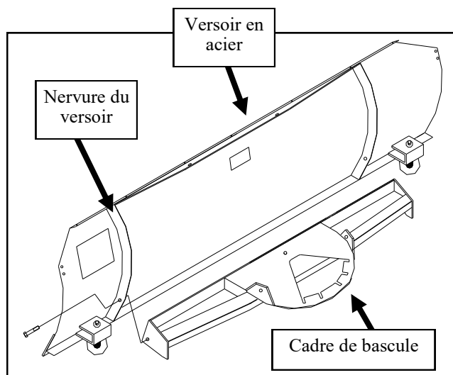
Figure 5.1— Fixation du cadre de bascule sur le versoir
