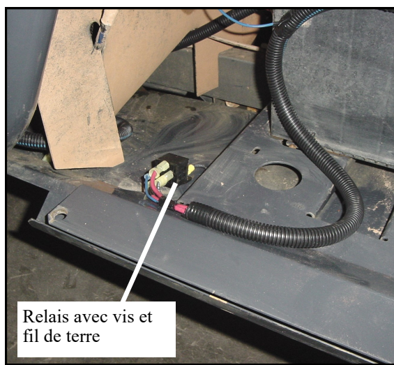
Photo 2 - Vue du côté gauche du RTV X900 avec le panneau latéral moulé retiré
