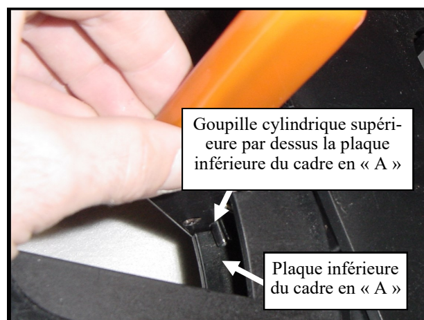
Figure 7.5—Poignée angulaire de lame
