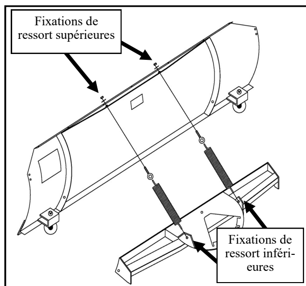
Figure 6.2— Installation des ressorts de bascule
