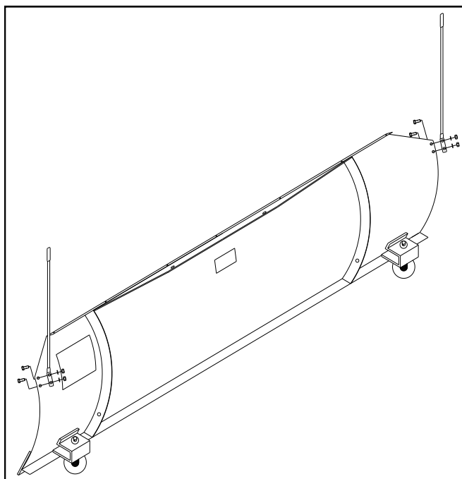
Figure 9.2—Installation du marqueur de lame
