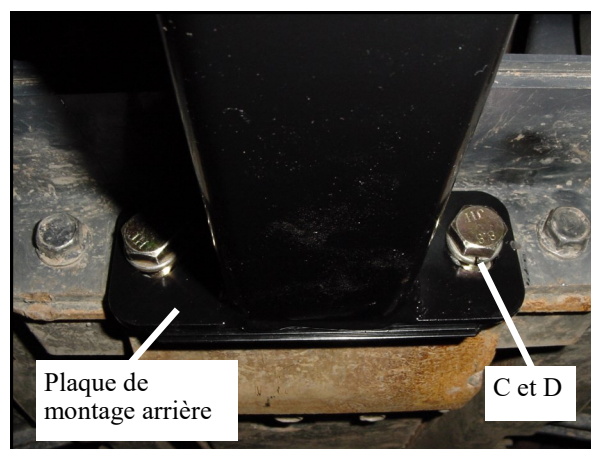
Montage de la plaque d'attelage arrière
